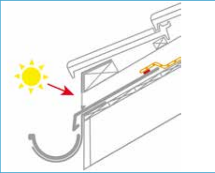
Raccord du pied de versant en cas de sollicitations extraordinaires. La sous-toiture est amenée directement dans la gouttière (veiller à protéger l'écran des UV au niveau du pied de versant !).
