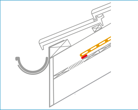
Raccord du pied de versant en cas de sollicitations normales et élevées.
