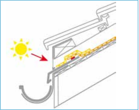
La sous-toiture est amenée directement dans la gouttière. Veiller à protéger l'écran des UV au niveau du pied de versant.
