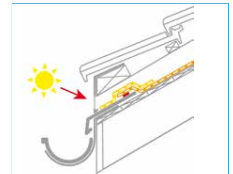
Das Unterdach wird direkt in die Rinne geleitet. UV-Schutz der Bahn im Traufbereich ist erforderlich.
