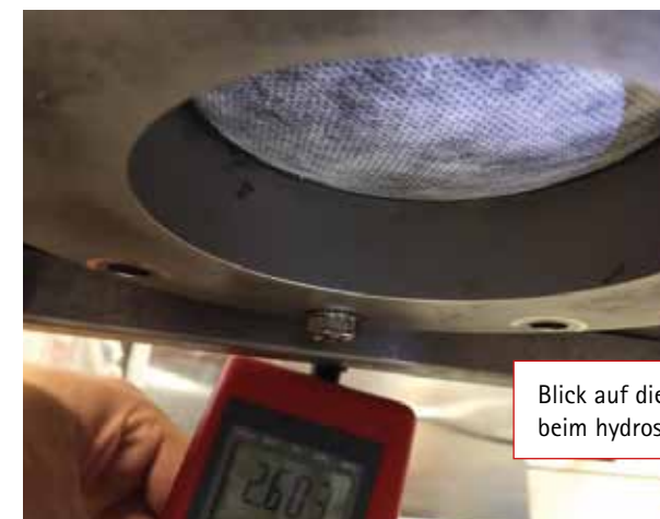
Hydrostatischer Drucktest mit einer SOLITEX MENTO 3000 nach fünf Jahren natürlicher Alterung unter Eindeckung – trocken bei 2.600 mm.
