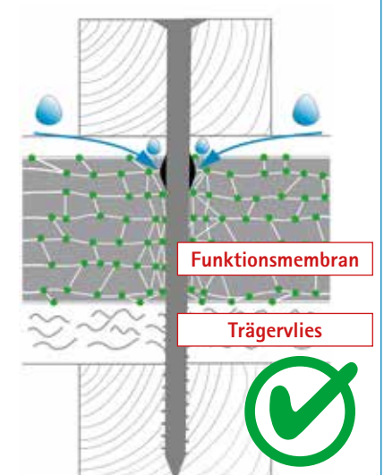
SOLITEX QUANTHO 3000 connect, Nageldichtung integriert mit porenfreier monolithischer TPU Funktionsmembran und Trägervlies
