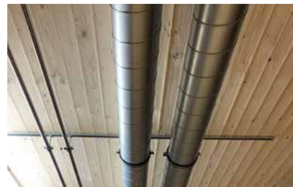
Überfeuchtete CLT-Decke
